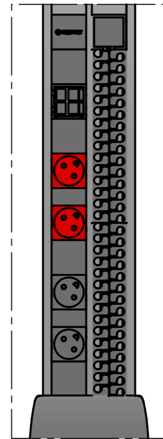
DETALLE A
